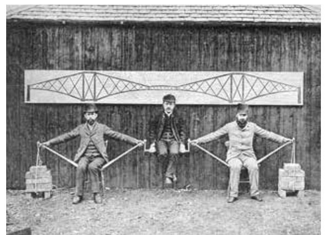
Die Ingenieure John Fowler, Kaichi Watanabe und Benjamin Baker demonstrieren das Prinzip des Einhängeträgers der Firth of Forth Bridge
